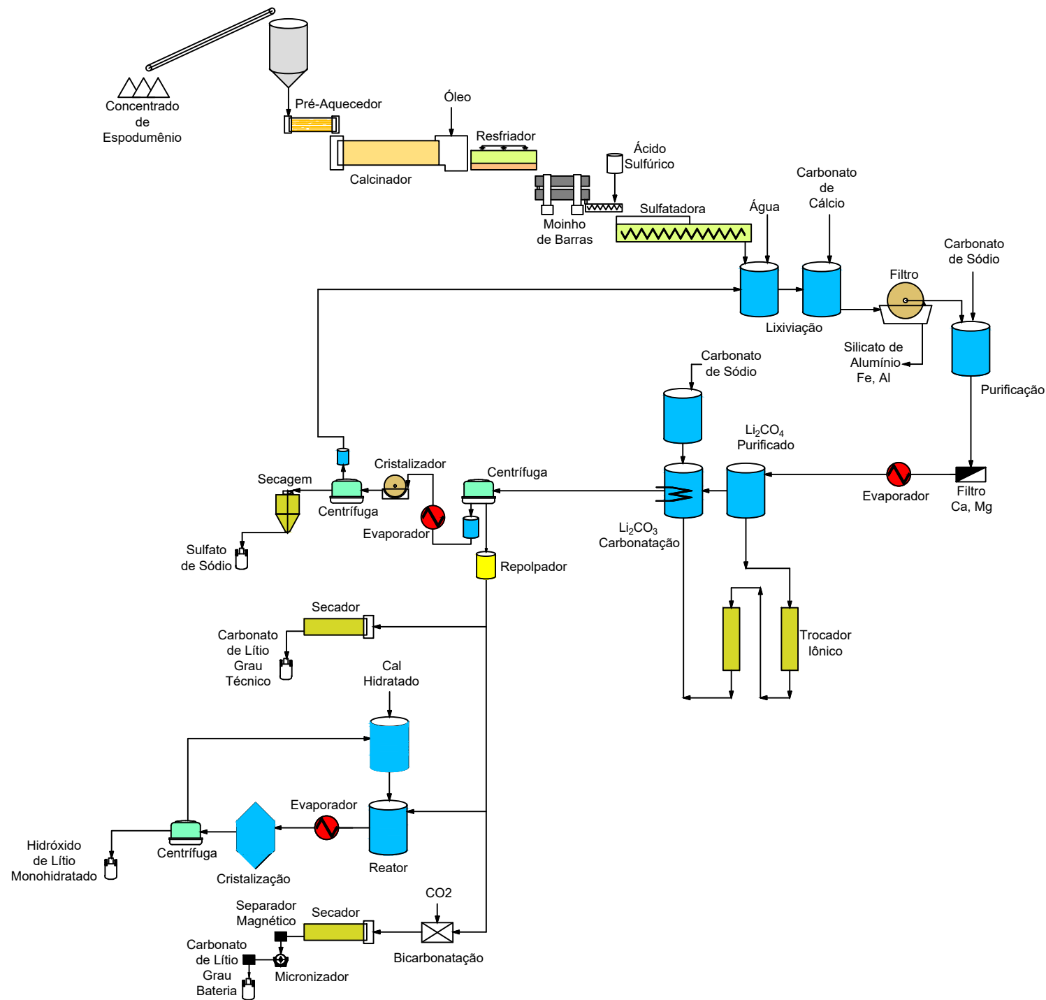
FLUXOGRAMA DE PROCESSO CBL PARA PRODUÇÃO DE CARBONATO DE LÍTIO GRAU BATERIA/GRAU TÉCNICO E HIDRÓXIDO DE LÍTIO GRAU TÉCNICO
